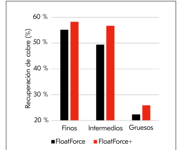
Recuperación de cobre en la primera celda de flotación rougher
