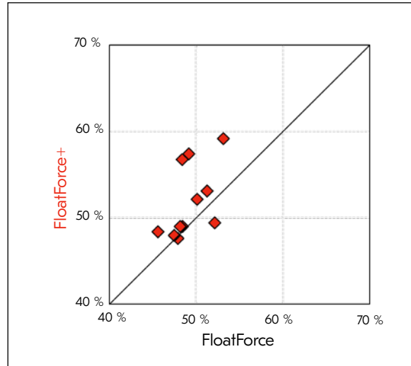
Recuperación de cobre con FloatForce+ y FloatForce
