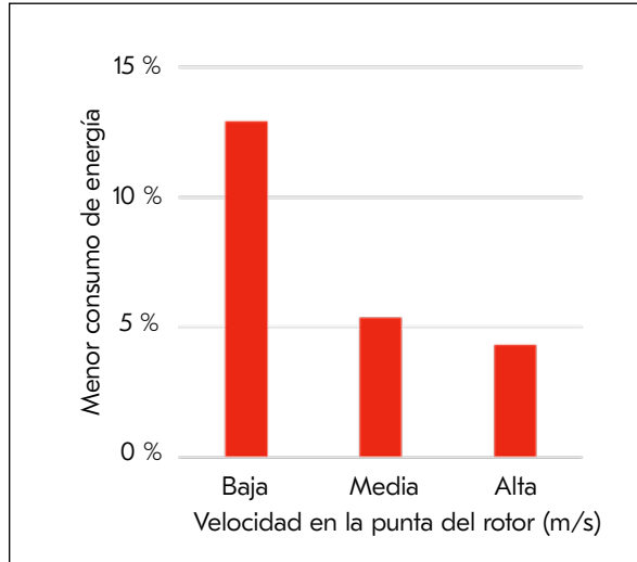
FloatForce+ vs. FloatForce a diferentes velocidades
